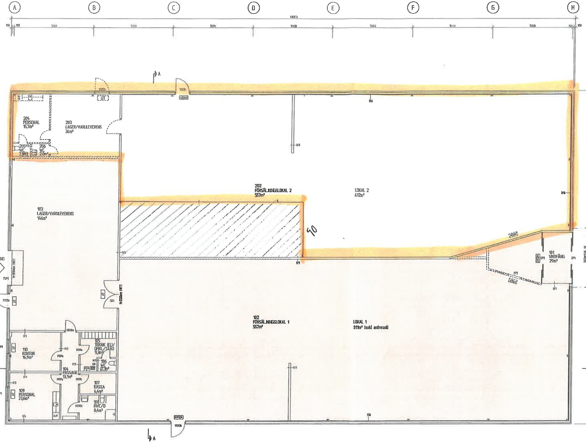
ENTRÉPLAN
