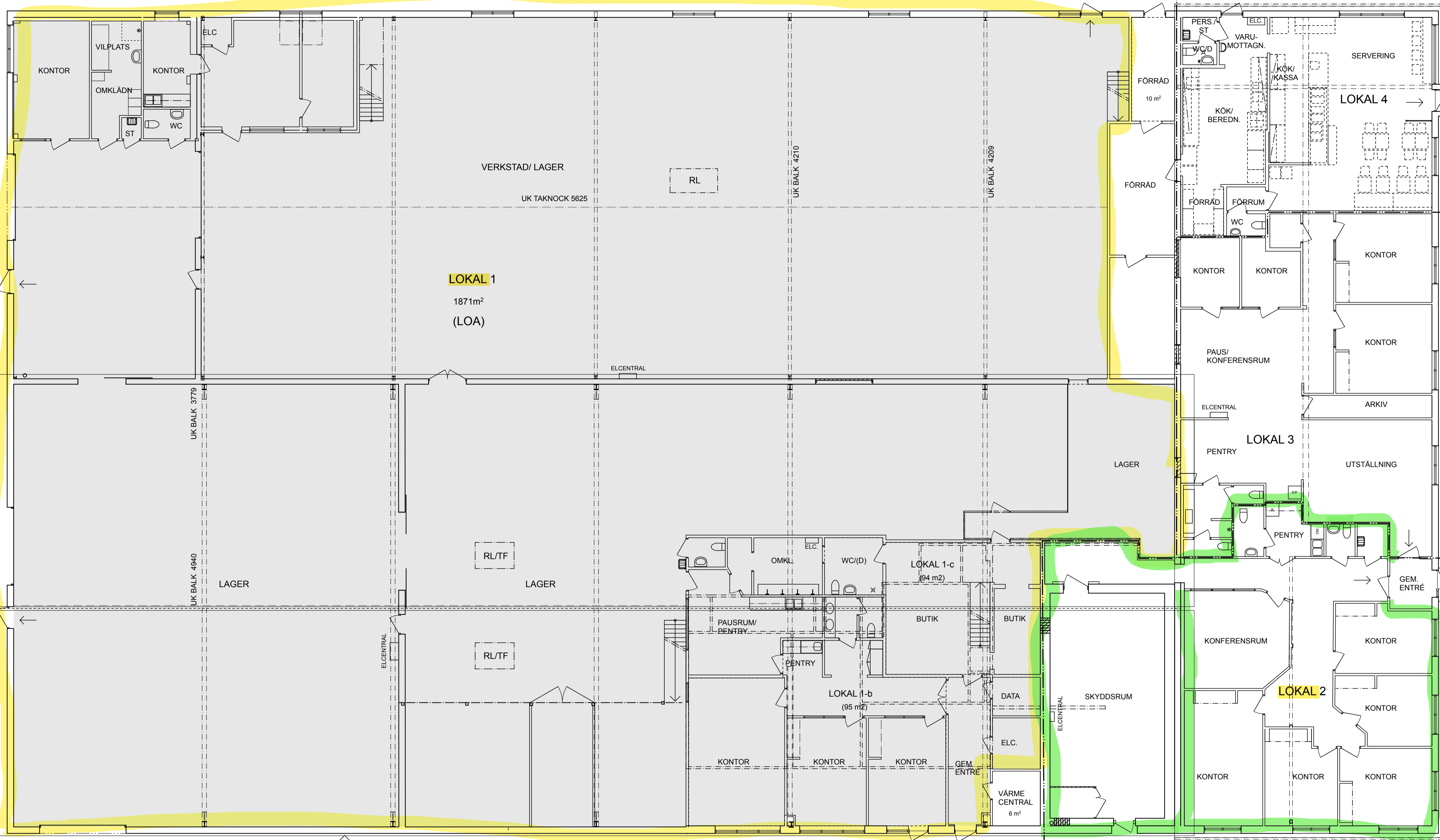
PLAN VÅNING 1 1:100 (A1)
